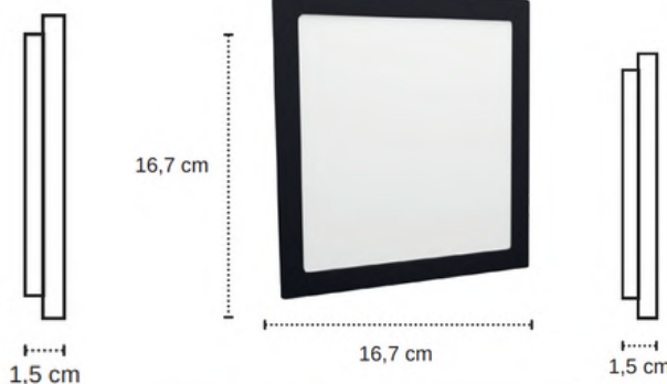
PAINEL SLIM DE EMBUTIR 18W MAXXY LED 3000K - cód. 5586 6500k - cód. 5583 1620 lumens
