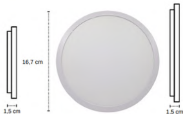
PAINEL SLIM DE EMBUTIR 12W MAXXY LED 3000K - cód. 5530 6500K - cód. 5407 1080 lumens
