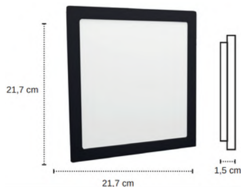
PAINEL SLIM DE EMBUTIR 24W MAXXY LED 3000K - cód. 5587 6500k - cód. 5584 2160 lumens
