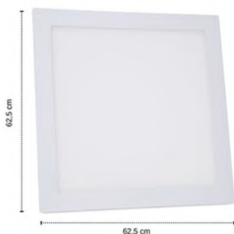
PAINEL SLIM DE EMBUTIR 48W MAXXY LED 4000K - cód. 5428 6500K - cód. 5403 3360 lumens
